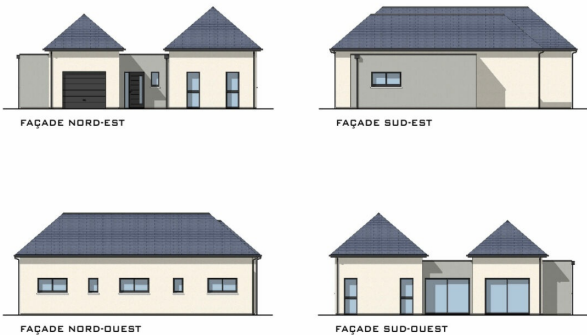
PLAN DES FAÇADES ET DES TOITURES
